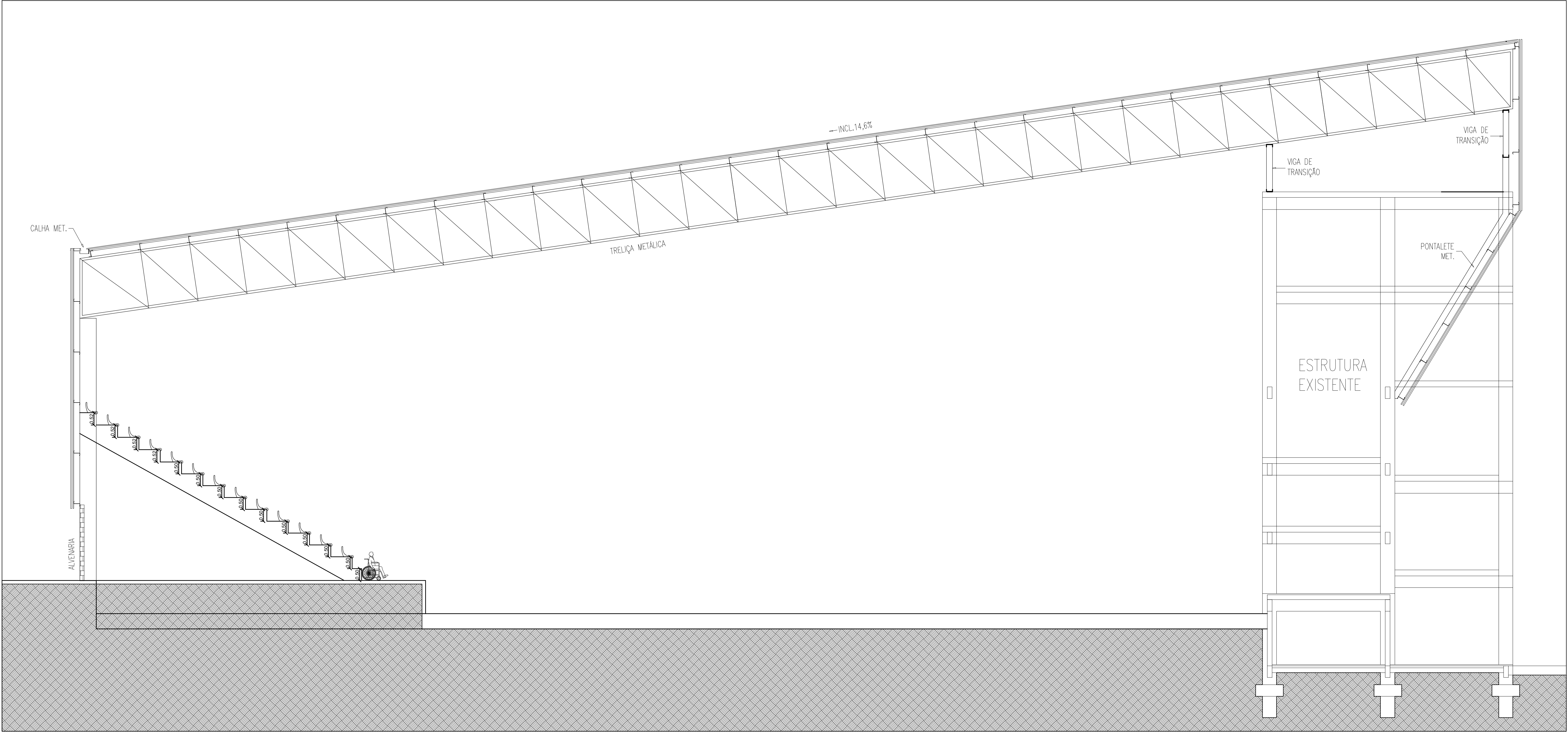
CORTE TRANSVERSAL EIXO 6
